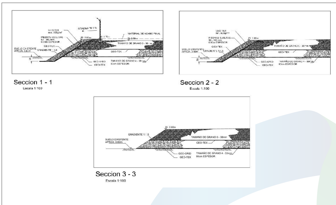
Figura 7. Secciones típicas del relleno.
