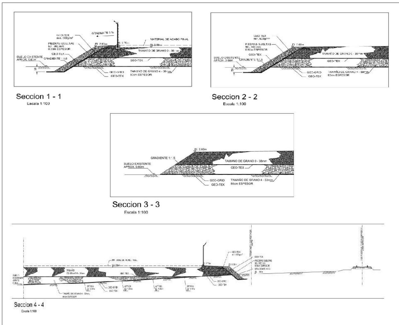
Figura 7. Secciones típicas del relleno.
